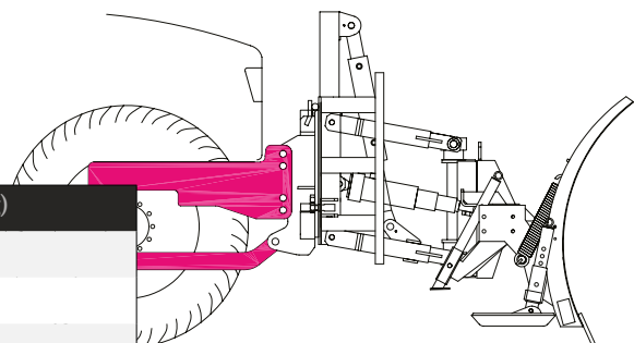
Montering av platen for kobling av snøpløgen
